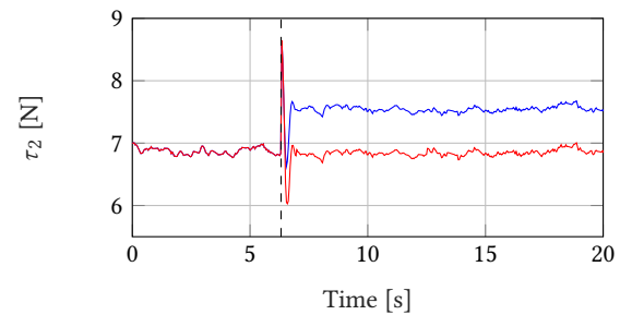
(d) Quadrotor 2 thrust command vs. experiment time.
